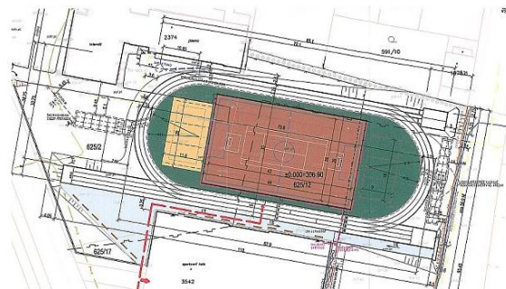
Plán školního hřiště
