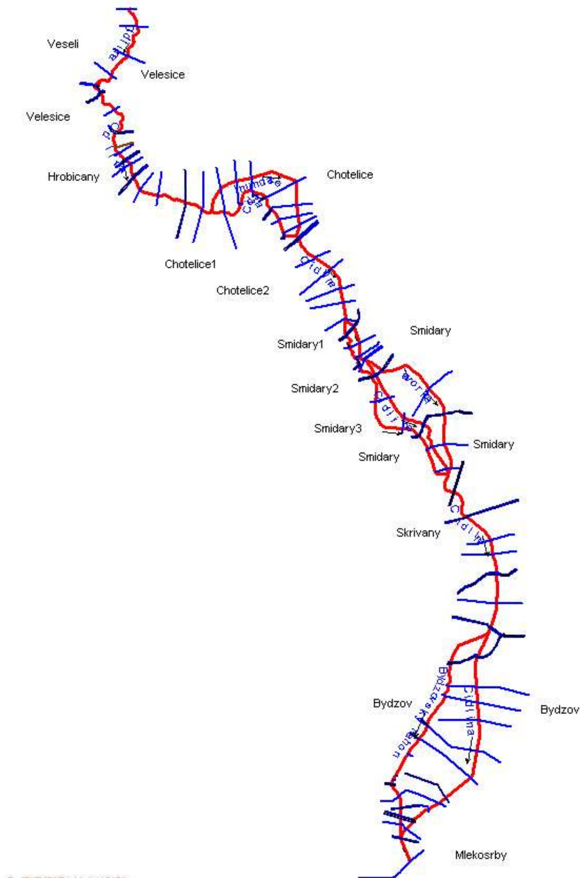
Obrázek 3 – Schéma hydraulického modelu Cidlina_II
