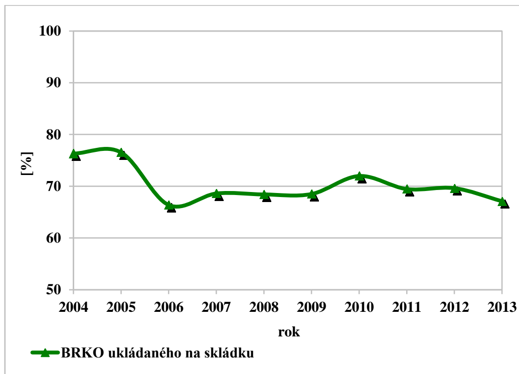
Graf 2.1.4i: Podíl BRKO ukládaného na skládky v letech 2004 – 2013 vzhledem ke srovnávací základně z roku 1995.
